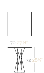
VERTEX Square Table 70 VERTEX Mesa Cuadrada 70
