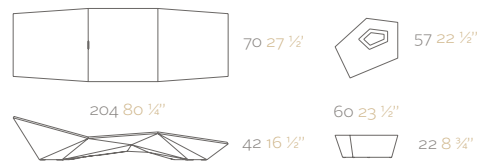
FAZ Sun Chaise FAZ Tumbona
