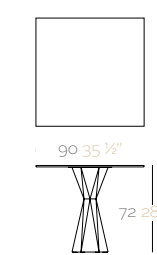
VERTEX Square Table 90 VERTEX Mesa Cuadrada 90
