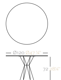
VERTEX Table Ø47 1/4" VERTEX Mesa Ø120
