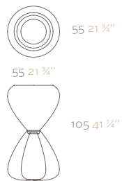
SPAGUETTI Pot Ø55 SPAGUETTI Maceta Ø55
