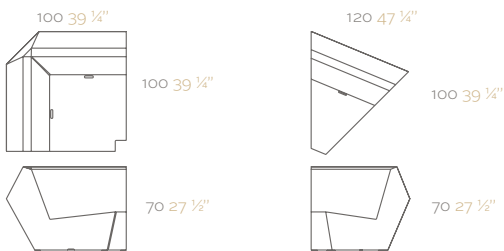
FAZ Sofa Corner 90° Unit FAZ Sofá Módulo Esquina 90°
