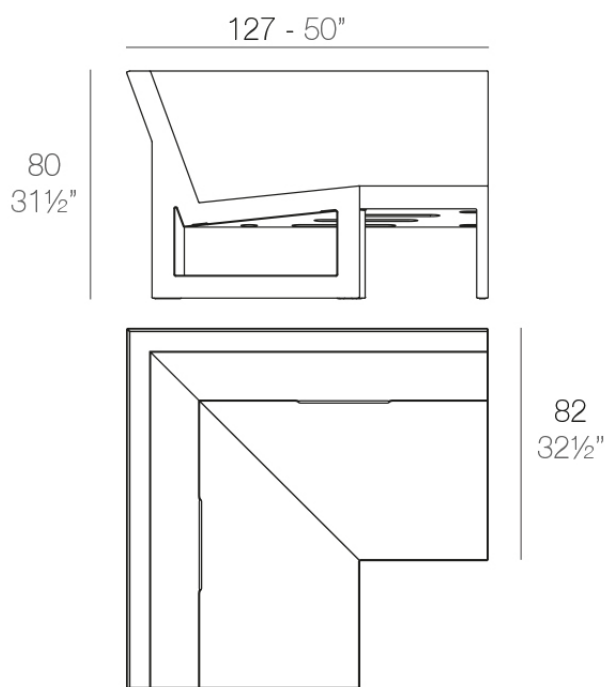
FRAME Sofá Módulo Esquina 90° FRAME Sectional Sofa Corner 90°
