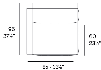
POSIDONIA Módulo derecho POSIDONIA Right armrest section
