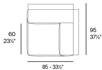
POSIDONIA Módulo esquina POSIDONIA Corner section
