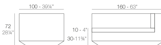
VELA Sofá Módulo Derecho Chaise Longue VELA Sectional Sofa Right Chaise Longue
