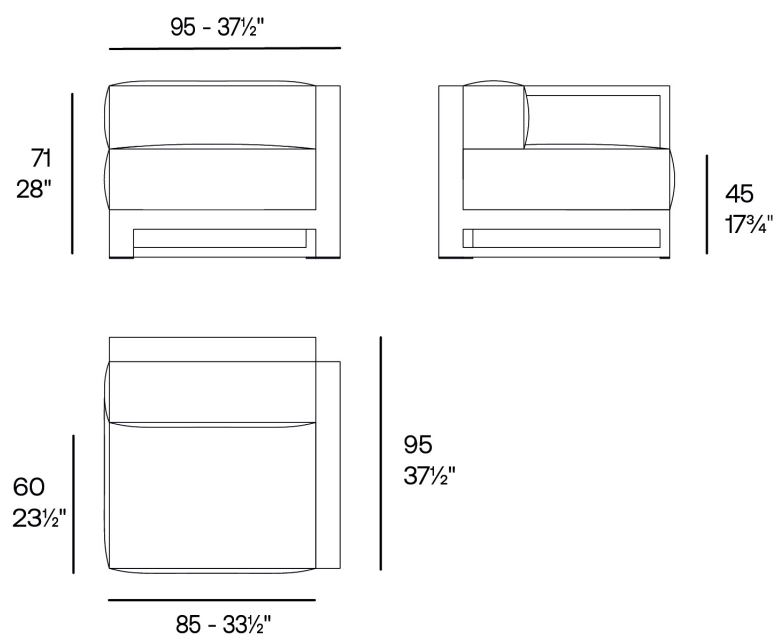
POSIDONIA Módulo izquierdo POSIDONIA Left armrest section
