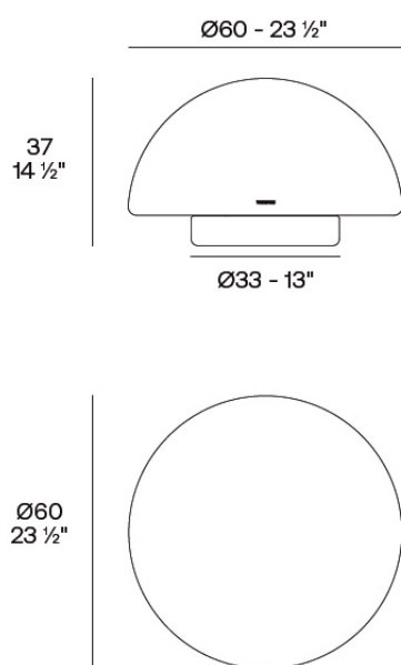
Luna. Lámpara Ø60x37 cm Luna. Lamp 23 1/2" x 14 1/2" 54860
