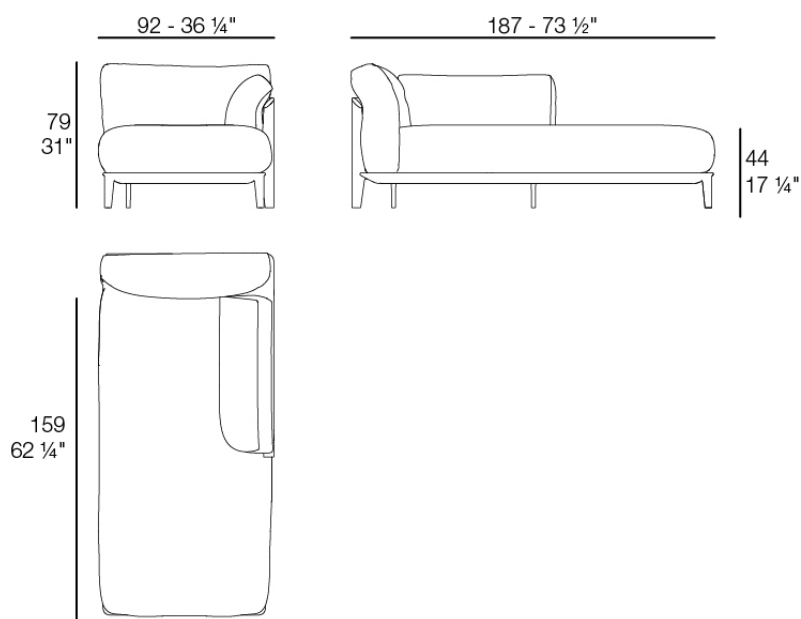
PASADENA Sofá Chaiselongue Izquierda PASADENA Sectional Sofa Chaiselongue Left Ref. 70059
